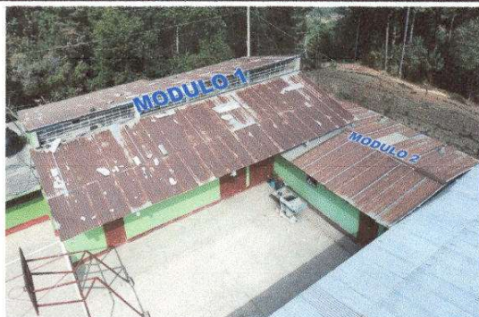
Foto 1: Sustitución de la lamina, por lamina troquelada color rojo calinre 26. 268 metros cuadrados en total.
